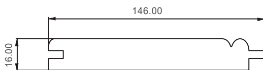
Altdeutsches Profil
