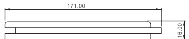
Rundfaseprofil-Short
