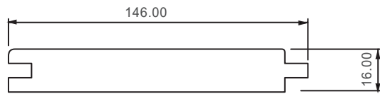
Swingprofil
