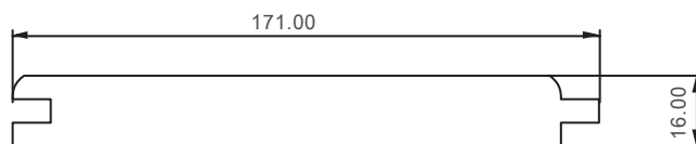
Rundfaseprofil
